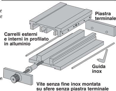
Carrello singolo DOMI50
