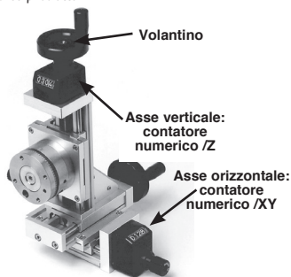
Slitte con volantini e contatori DOMI50-CV (esempio d'applicazione)
