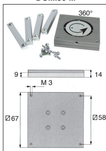
Piatto girevole DOMI 50-PT
