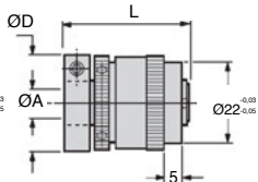
VT4 con ganascia di serraggio
