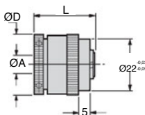
VT2 Con vite a pressione
